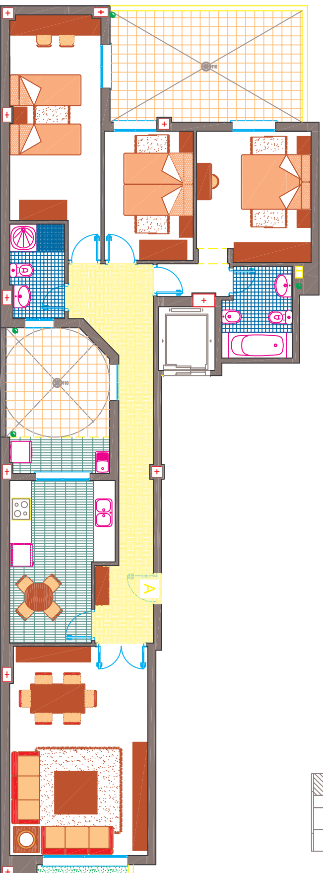
VIVENDA TIPUS A PLANTA BAIXA
